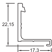
Section No. RB-230 17.3mm Hook Bead 0.148kg/m, per 86
