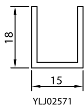
YLJ02571
