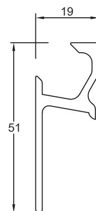
Section No. RB-260 0.522 kg/m, per 162
