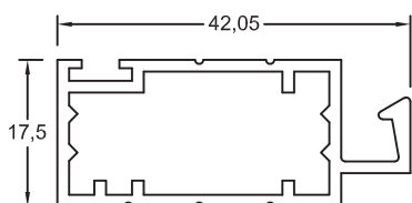
Section No.9775 Door Frame 0.494kg/m, per 260
