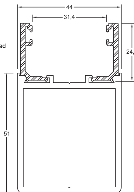
Section No. 5622 Hinge Stile 1.299kg/m, per 215
