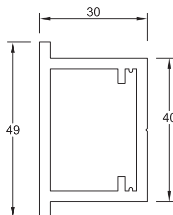
Section No.RB-842 1.170 kg/m, per 158
