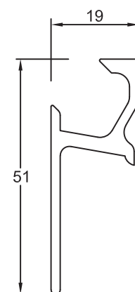
Section No. RB-260 0.522 kg/m, per 162
