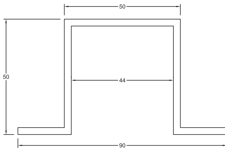
Section No. RB-854 1.490kg/m, per 374
