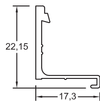
Section No.RB-230 17.3mm Hook Bead 0.148kg/m, per 86
