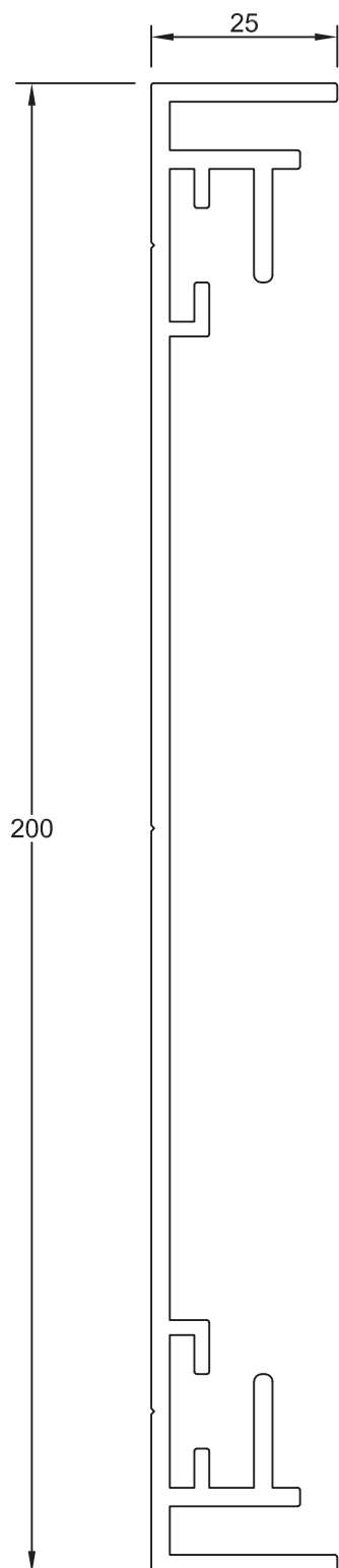
Section No.36166 2.270 kg/m, per 686
