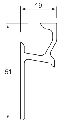
Section No.RB-260 0.522 kg/m, per 162
