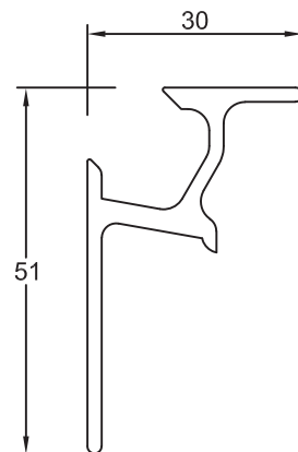
Section No.RB-286 0.587 kg/m, per 182
