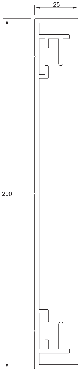
Section No.36166 2.270 kg/m, per 686
