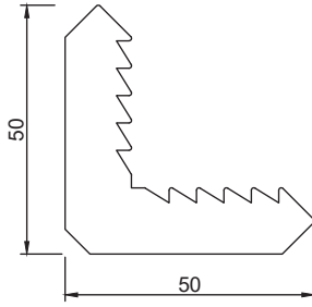
Section No. X124 2.667 kg/m, per 218
