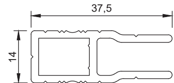
Section No. G253 0.500 kg/m, per 147
