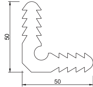
Section No. 6180A 2.379 kg/m, per 267
