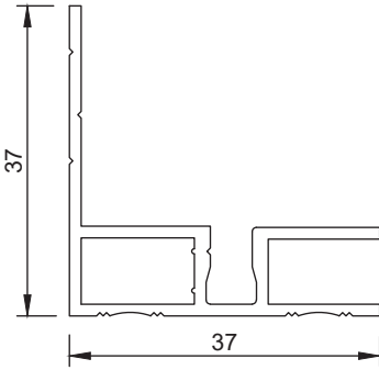
Section No. RB-123 0.454 kg/m, per 198
