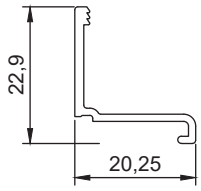
Section No. E771 0.159 kg/m, per 89.6
