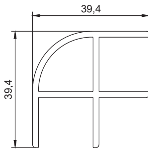
Section No. 30505 0.764 kg/m, per 280.6
