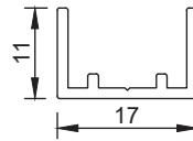
*Section No.31018 0.139 kg/m, per 81
