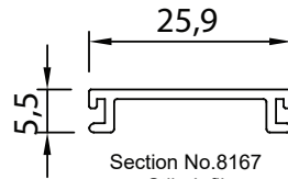
Section No. 8167 Stile Infil 0.140 kg/m, Per 85
