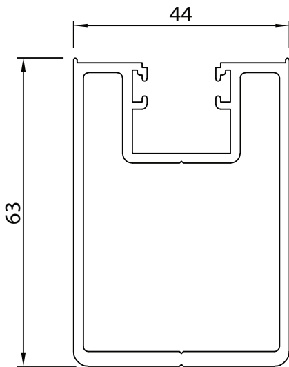
Section No. G250 Hinge Stile 1.470 kg/m, Per 286
