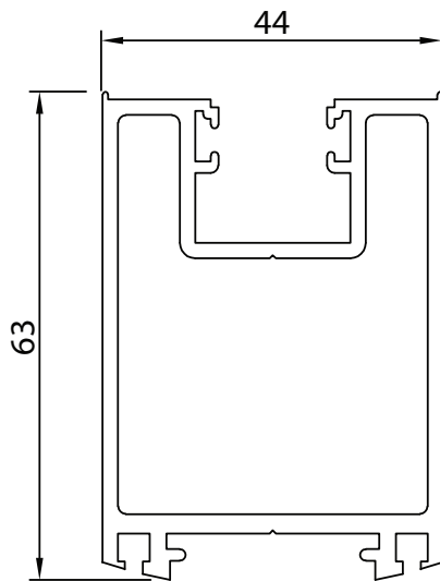
Section No. G249 Lock Stile 1.510 kg/m, Per 331
